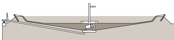
Sezione del prodotto Alligator Bagtank vuoto.
