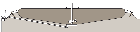
Sezione del prodotto Alligator Bagtank pieno.
